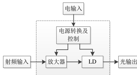
图 1 产品工作原理框图
